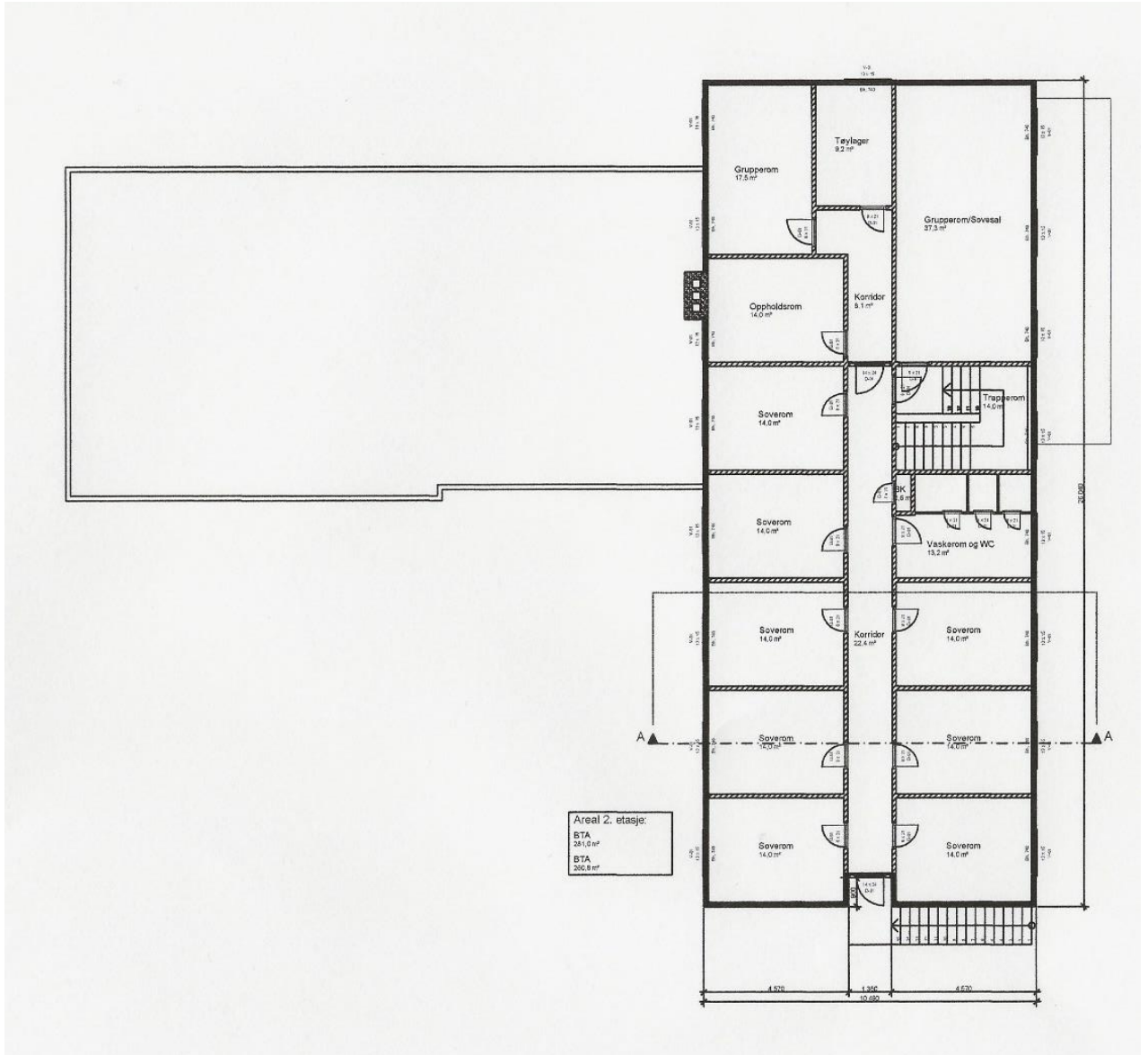
Andre etasje
